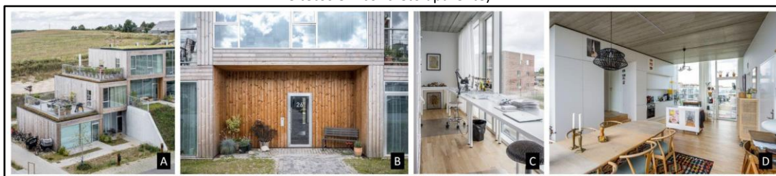
Figura 9 – Fotografias do Edifício Residencial Sneglehusene (A: Imagem externa, mostrando os módulos em concreto revestidos em madeira, alguns terraços e telhados verdes. B: Imagem externa, mostrando os revestimentos em madeira e fechamentos com vidros duplos. C e D: Imagens internas, mostrando pisos em madeira e tetos em concreto aparente).
