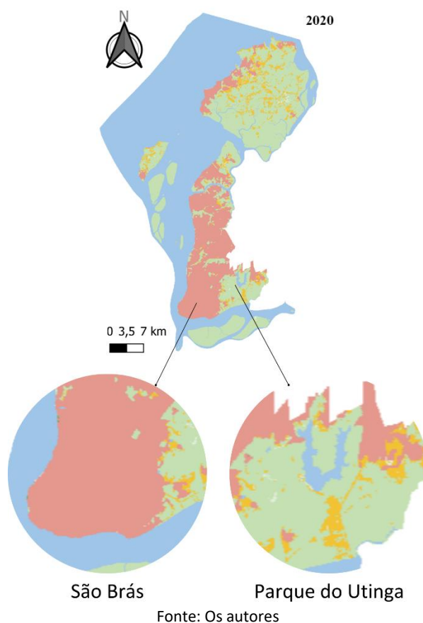
Figura 3: Imagens da classe do uso e cobertura do solo do entorno das estações meteorológicas, bairro de São Brás e Parque do Utinga.
