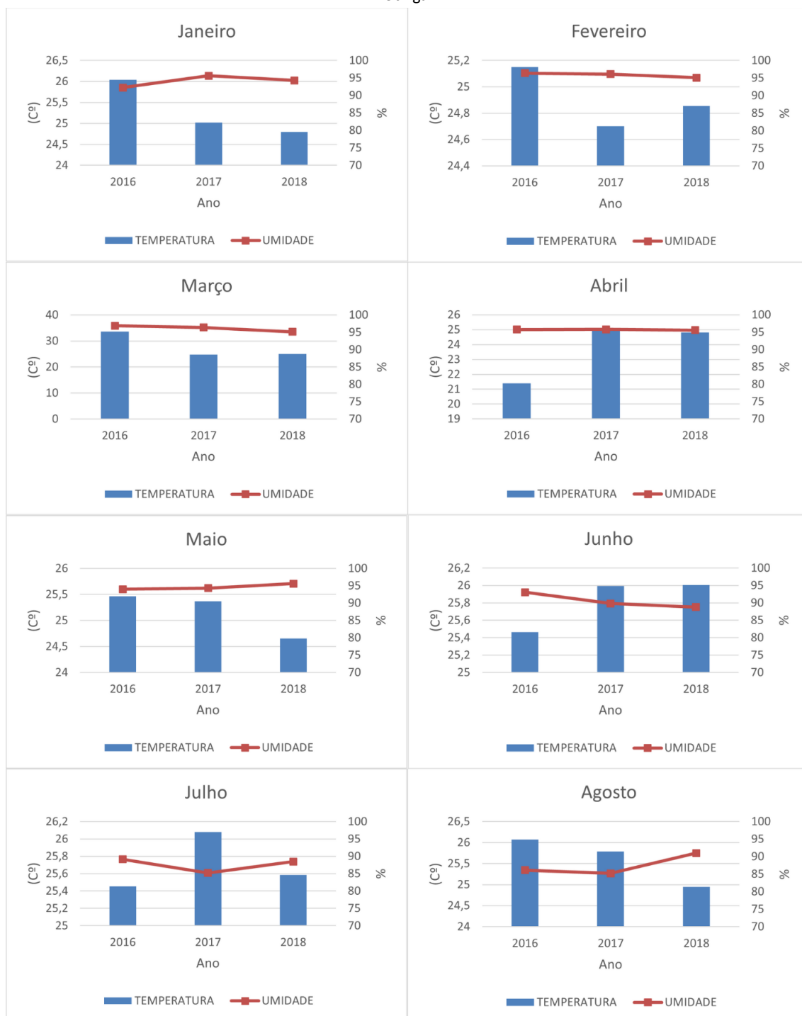
Figura 4: Temperatura e umidade relativa média dos anos de 2016 e 2018 da estação meteorológica do Parque do Utiga.
