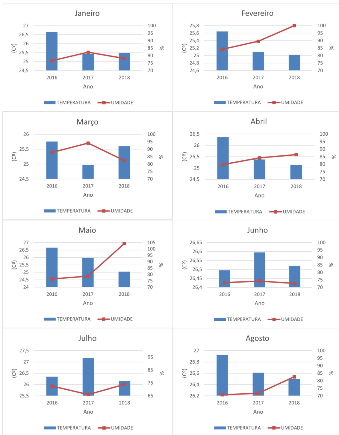
Figura 5: Temperatura e umidade relativa média dos anos de 2016 e 2018 da Estação meteorológica do Bairro de São Braz.
