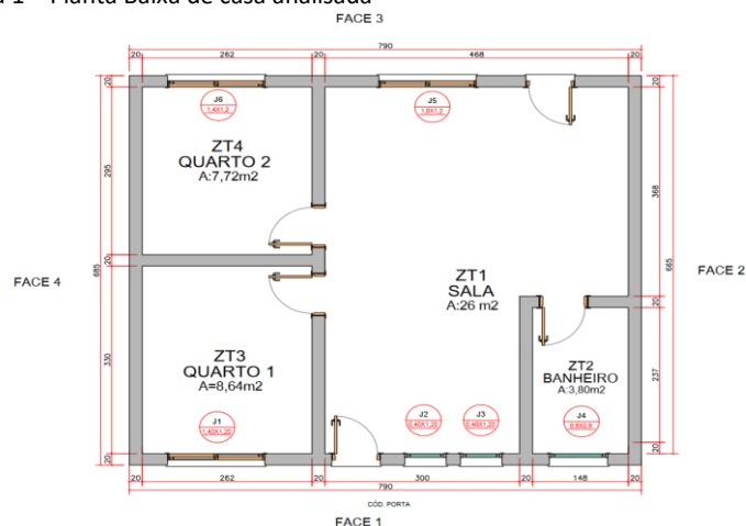
Figura 1 – Planta Baixa de casa analisada
