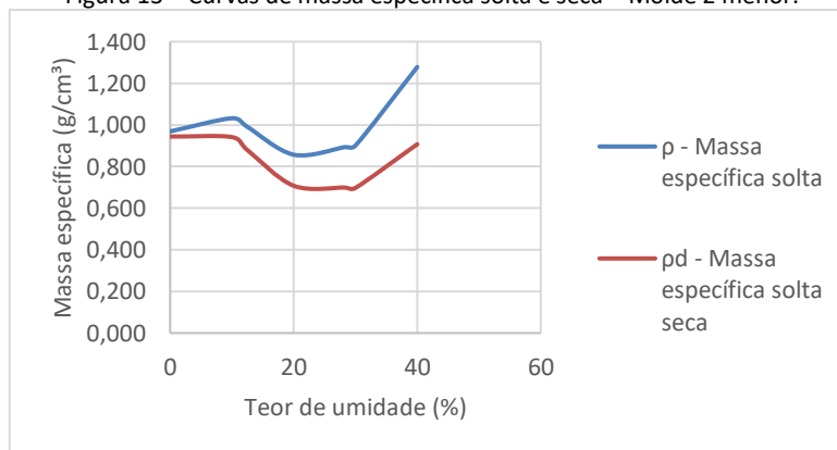
Figura 13 – Curvas de massa específica solta e seca – Molde 2 menor.
