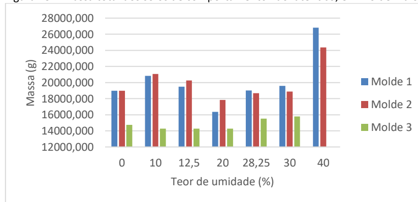
Figura 15 – Massa total dos solos de comportamento não laterítico, em molde maior.
