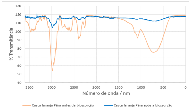
Gráfico 5: Espectro infravermelho da casca da laranja Pêra
