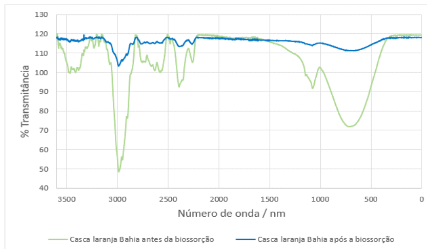
Gráfico 7: Espectro infravermelho da casca da laranja Bahia
