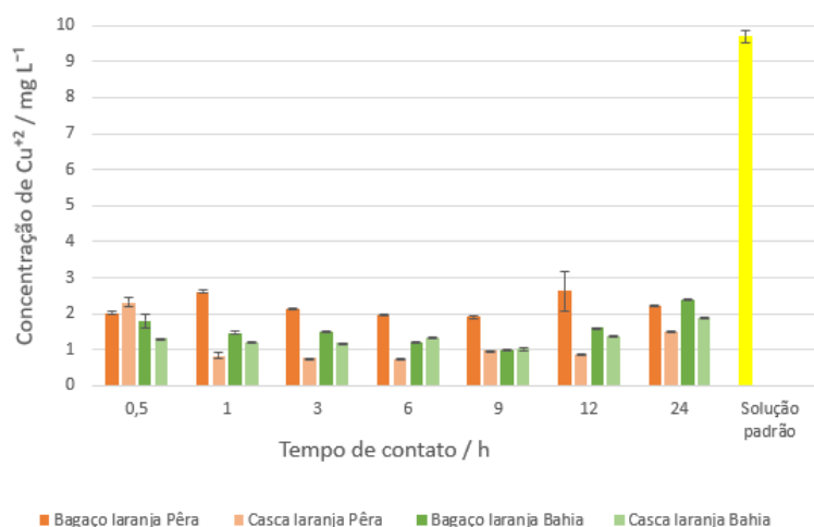
Gráfico 2: Investigação do tempo de contato entre solução metálica e bio sorventes
