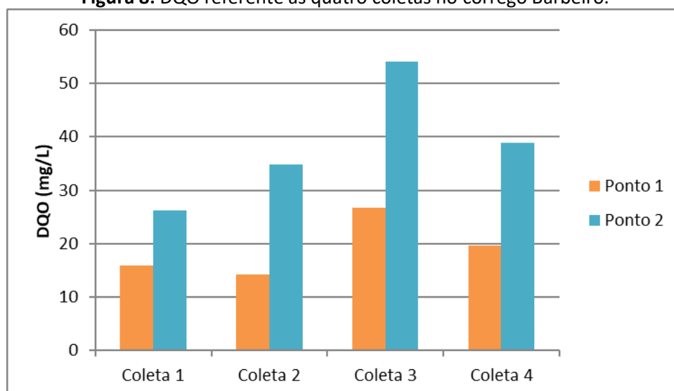
Figura 8: DQO referente as quatro coletas no córrego Barbeiro.
