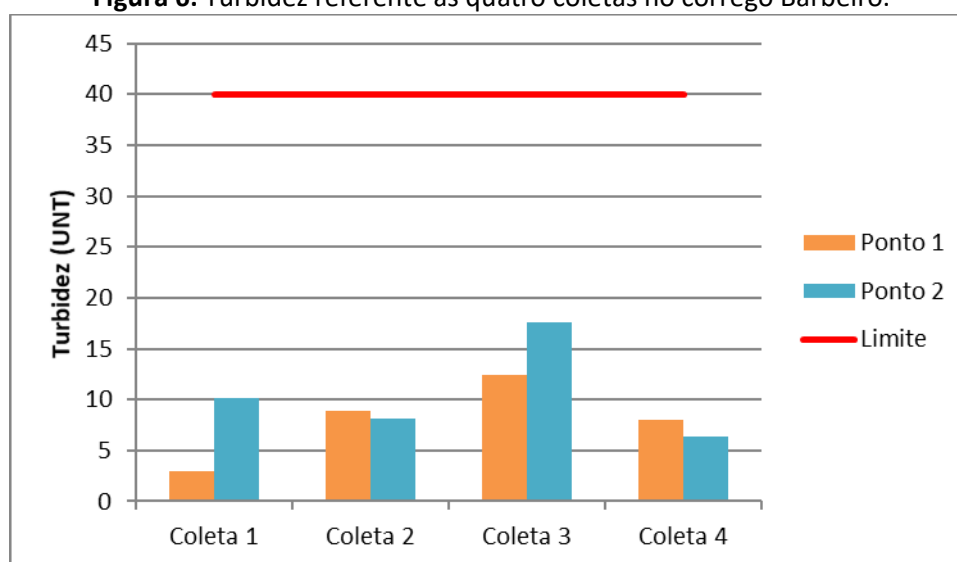
Figura 6: Turbidez referente as quatro coletas no córrego Barbeiro.
