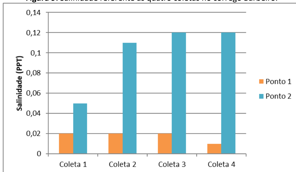
Figura 9: Salinidade referente as quatro coletas no córrego Barbeiro.
