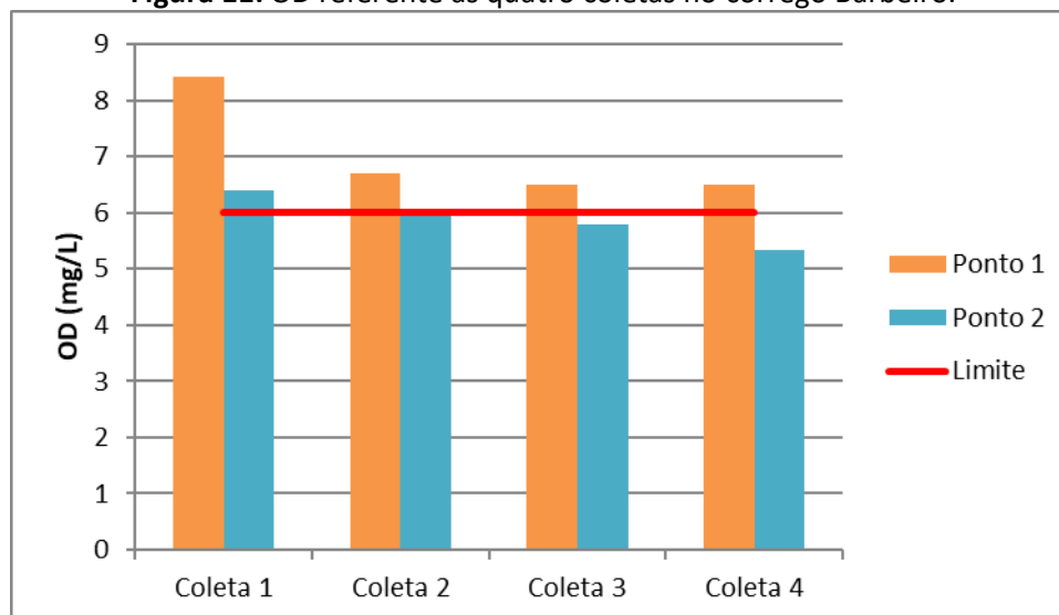
Figura 11: OD referente as quatro coletas no córrego Barbeiro.
