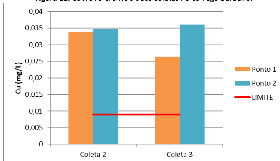
Figura 12: Cobre referente a duas coletas no córrego Barbeiro.
