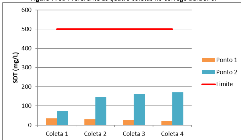
Figura 7: SDT referente as quatro coletas no córrego Barbeiro.
