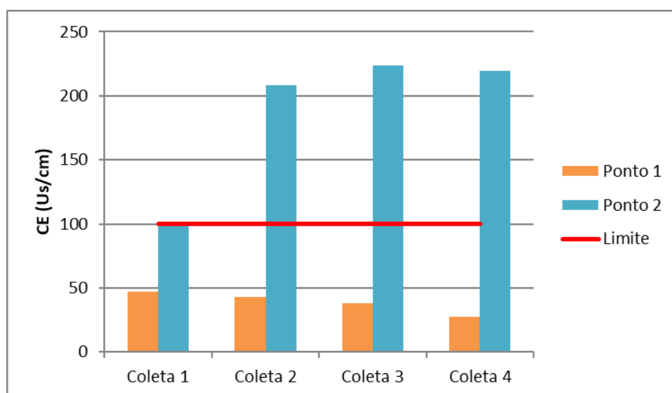
Figura 10: CE referente as quatro coletas no córrego Barbeiro.
