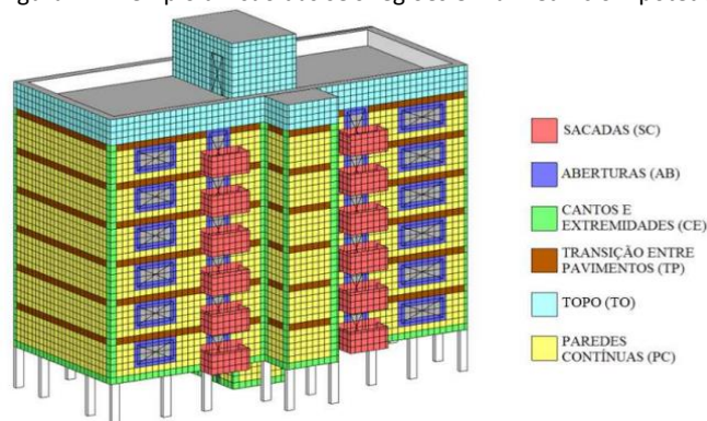
Figura 4 - Exemplo divisão das seis regiões em um edifício hipotético
