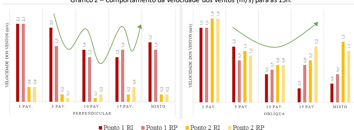
Gráfico 2 – Comportamento da velocidade dos ventos (m/s) para às 15h.
