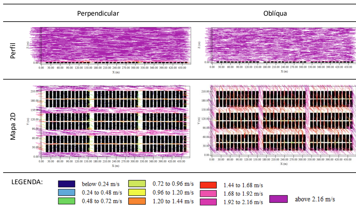
Quadro 4 - Perfis e mapas de ventilação, modelo REF de incidência da ventilação perpendicular e oblíqua.
