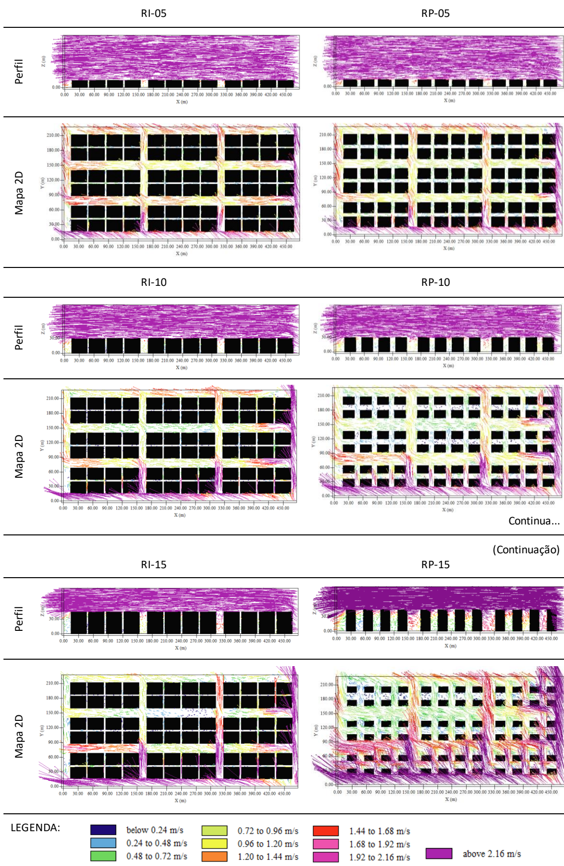
Quadro 6 - Perfis e mapas de ventilação às 15h, de incidência da ventilação oblíqua às edificações (N=45°).
