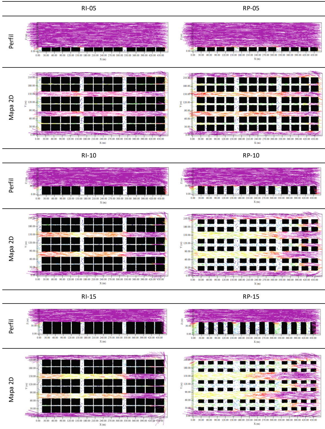
Quadro 5 - Perfis e mapas de ventilação às 15h, de incidência da ventilação perpendicular às edificações (N=0°).
