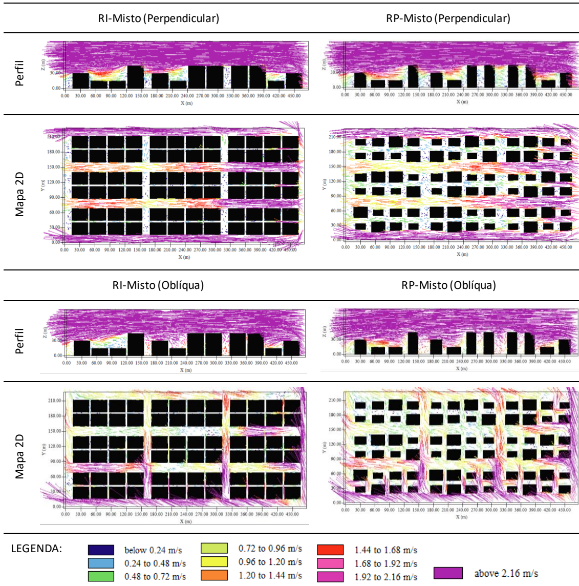
Quadro 7 - Perfis e mapas de ventilação às 15h, de incidência da ventilação perpendicular e oblíqua.
