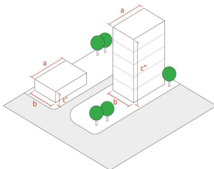
Figura 1 - Esquema de dimensionamento do fluxo de escoamento superficial em coberturas e fachadas Escoamento Superficial ( Q_{max} ) = Intensidade de Precipitação ( I_m ) x Área ( A ) x ...
