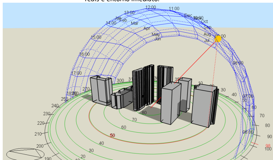
Figura 1 – Perspectiva isométrica do edifício modelado no software DesignBuilder com coordenadas reais e entorno imediato.
