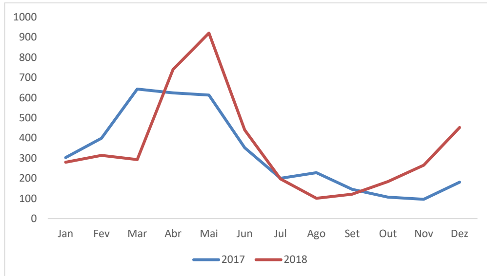
Figura 2- Sazonalidade dos casos de Dengue, por mês, entre 2017-2018, em Uberlândia (MG).
