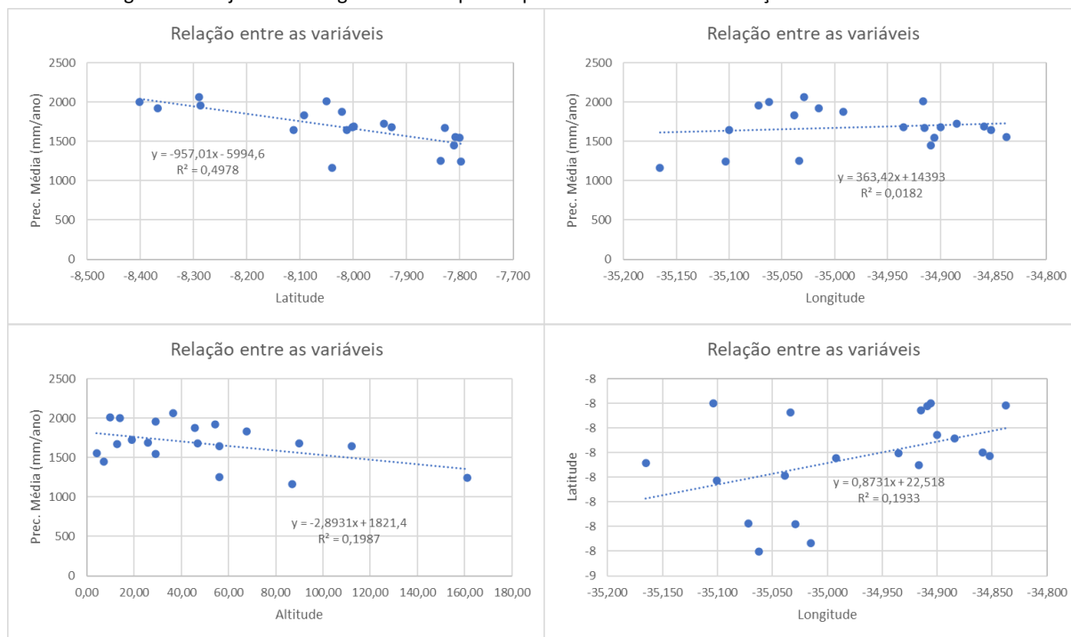
Figura 3 – Conjunto de Diagramas de Dispersão para Analisar Possíveis Relações entre as Variáveis
