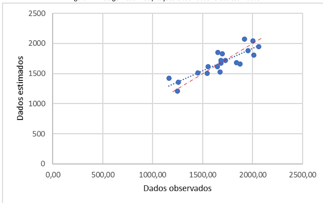
Figura 4 – Plotagem das Precipitações Observadas versus estimadas
