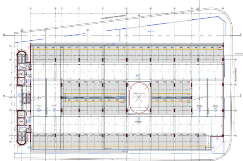
Figura 3 – Planta baixa de um pavimento do edifício garagem
