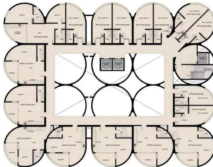
Figura 5 – Planta baixa do pavimento tipo do edif, Silo 215
