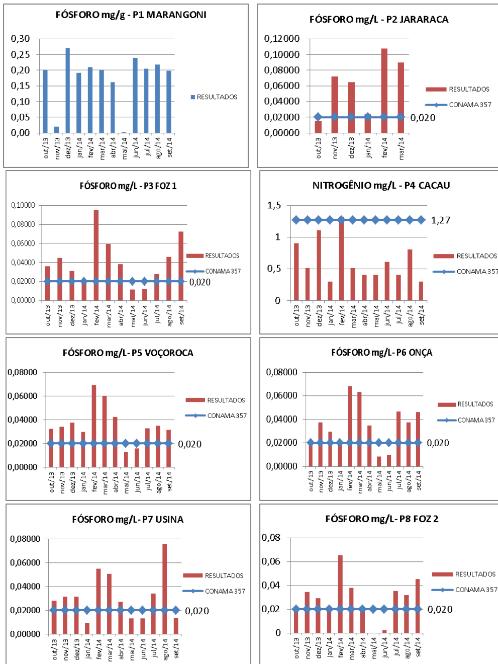
Figura 3: Resultados do parâmetro Fósforo em todos os pontos de coleta da Microbacia
