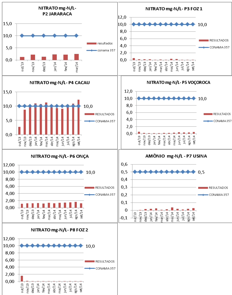
Figura 6: Resultados do parâmetro Nitrato em todos os pontos de coleta da Microbacia
