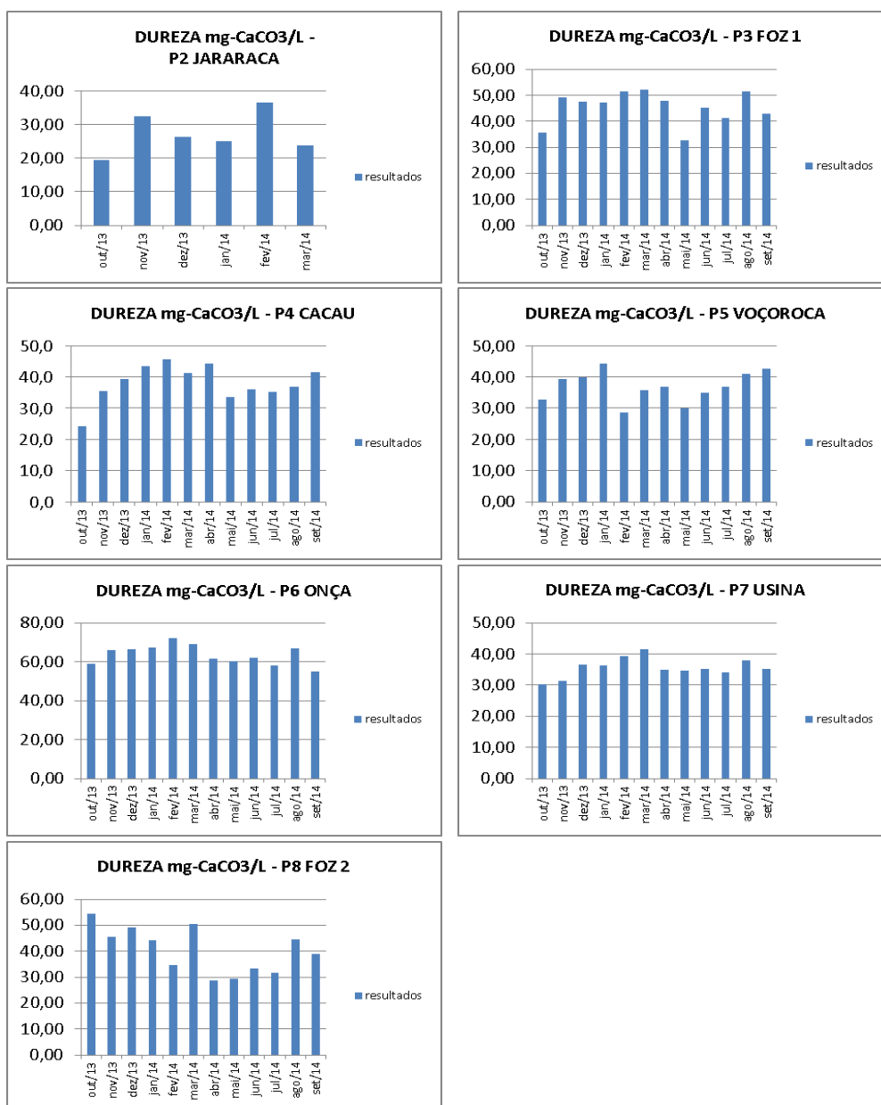
Figura 4: Resultados do parâmetro Dureza em todos os pontos de coleta da Microbacia
