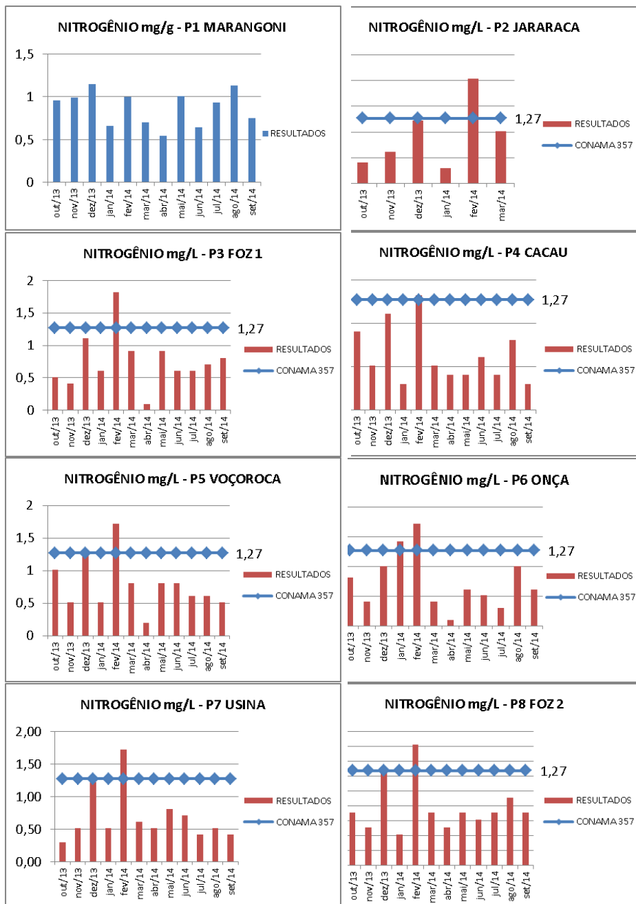
Figura 2: Resultados do parâmetro Nitrogênio em todos os pontos de coleta da Microbacia
