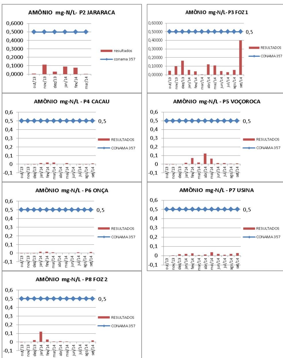
Figura 5: Resultados do parâmetro Amônio em todos os pontos de coleta da Microbacia
