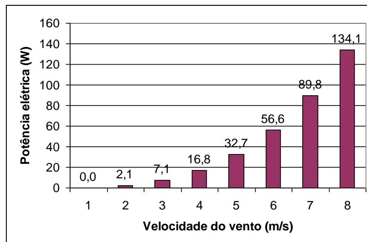
Figura 11. Potência elétrica.
