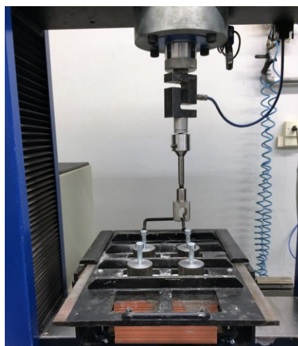
Figura 1 : Ensaio de resistência de aderência
