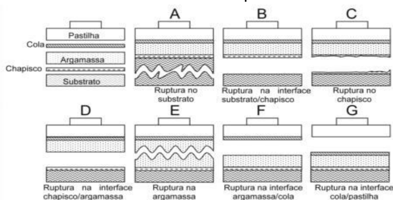
Figura 2- Formas de ruptura no ensaio de resistência de aderência à tração para um sistema de revestimento com chapisco
