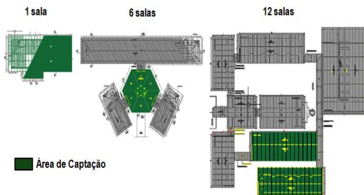
Figura 3 - Área de Captação por tipologia predial para Caruaru e Petrolina.
