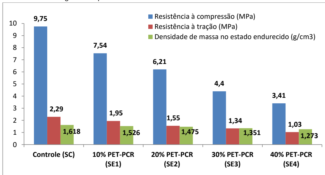
Figura 2: Propriedades mecânicas: Densidade de massa e resistências
