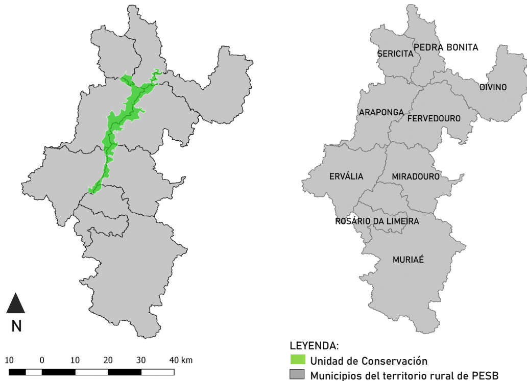
Figura 03. Localización de la Unidad de Conservación del Parque Estatal de la Serra do Brigadeiro y municipios.
