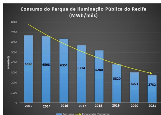
Figura 2 - Gráfico de previsão de consumo após substituição das luminárias da cidade por LED.
